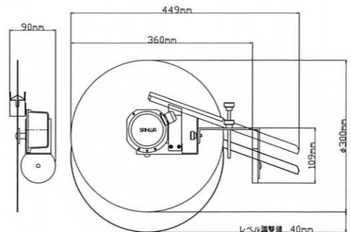
■スタンダードタイプ応用取付例
